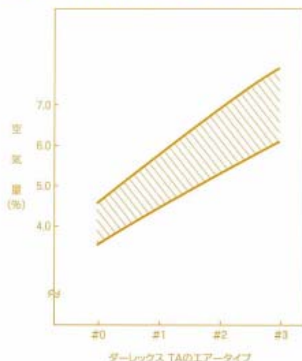
エアータイプ(# )と空気量の関係
